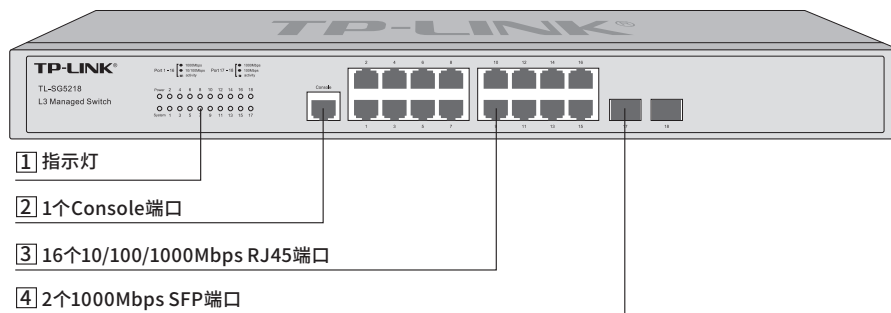
图1-4 TL-SG5218前面板示意图
