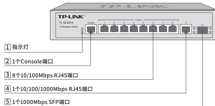
图1-9 TL-SL5210前面板示意图
