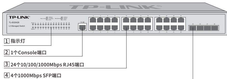
图1-2 TL-SG5428前面板示意图
