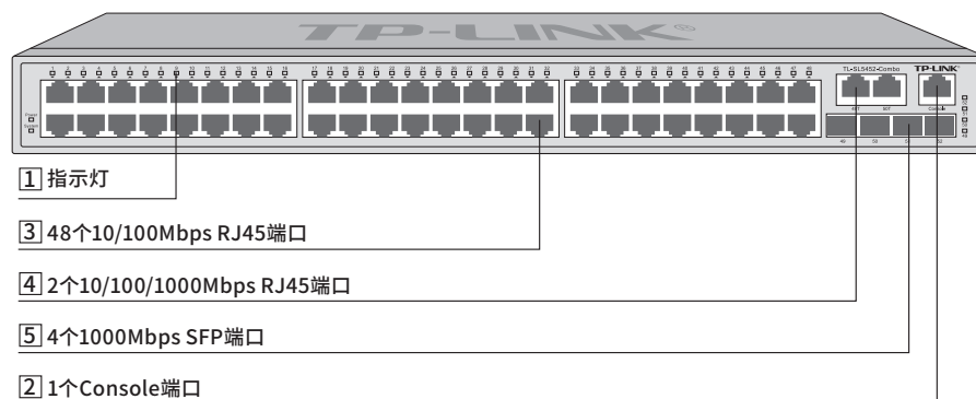
图1-6 TL-SL5452-Combo前面板示意图
