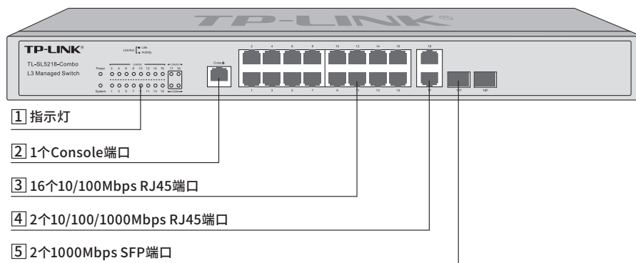
图1-8 TL-SL5218-Combo前面板示意图
