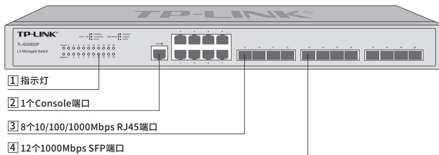
图1-3 TL-SG5820F前面板示意图
