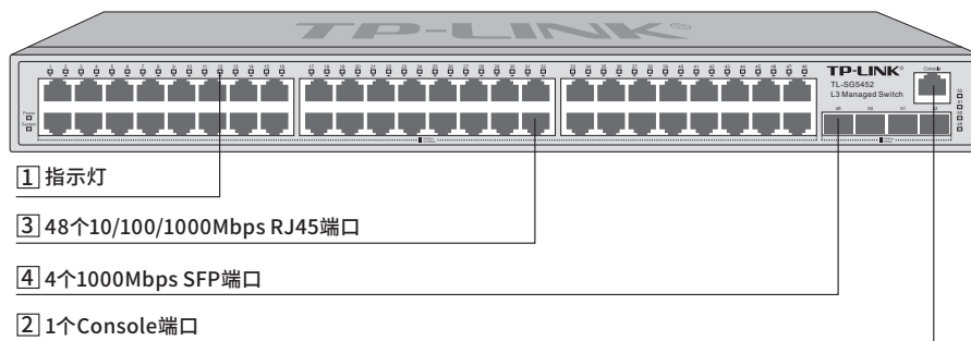
图1-1 TL-SG5452前面板示意图
