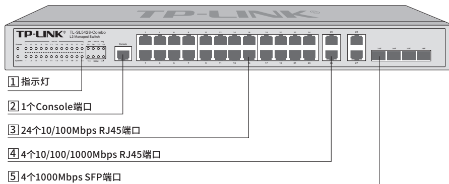
图1-7 TL-SL5428-Combo前面板示意图
